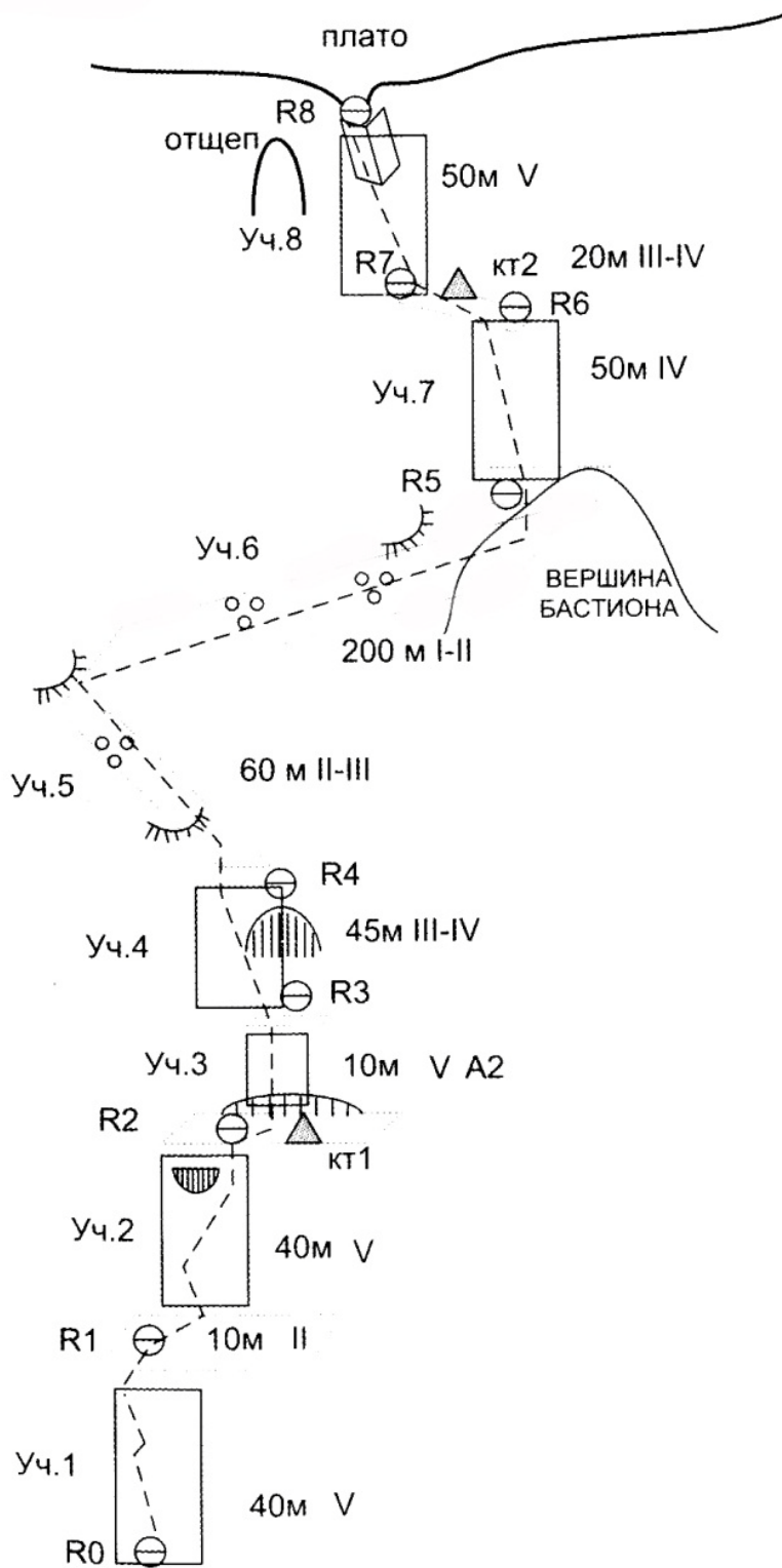
Рис. 3. Схема UIAA.
