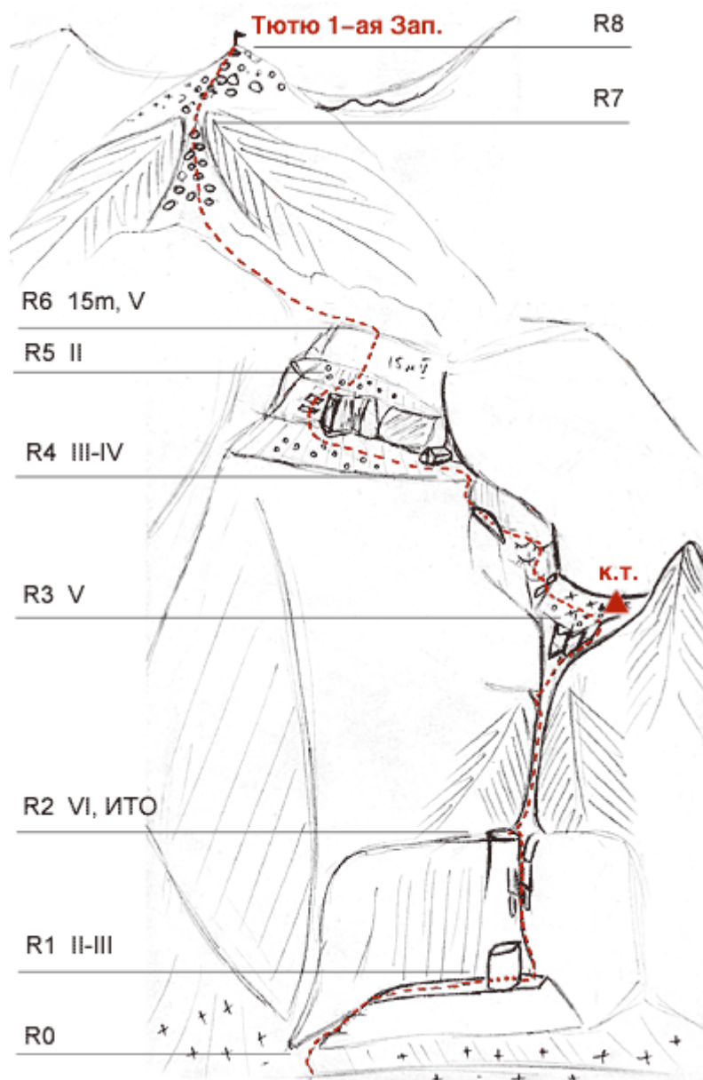
Рис. 2. Схема маршрута в символах УИАА
