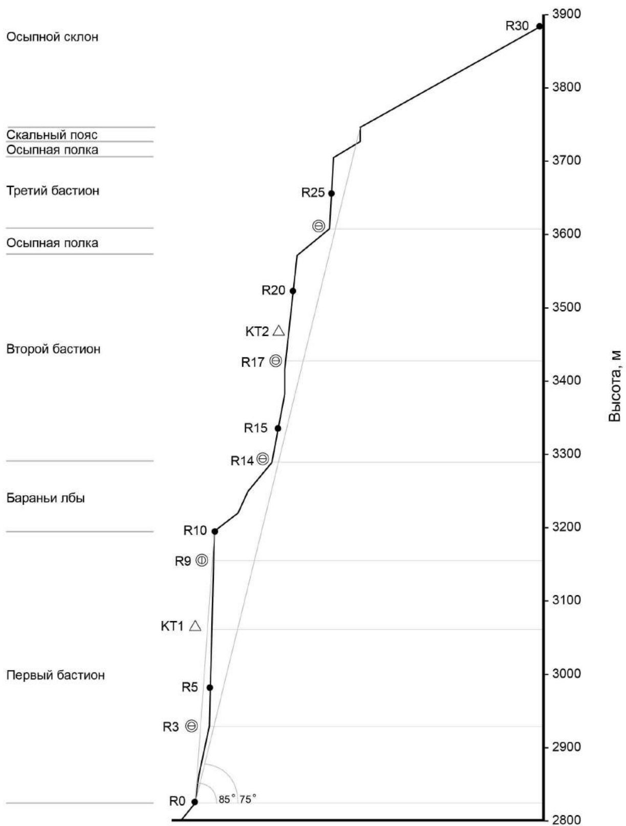
Рис. 1 Профиль стены массива Ерыдаг в месте расположения маршрута
