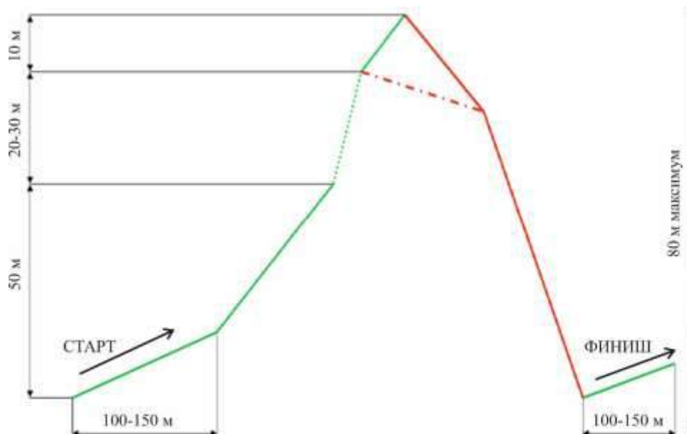
Профиль трассы
